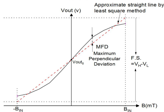
图 1. HAL4401-SR8输出特性
