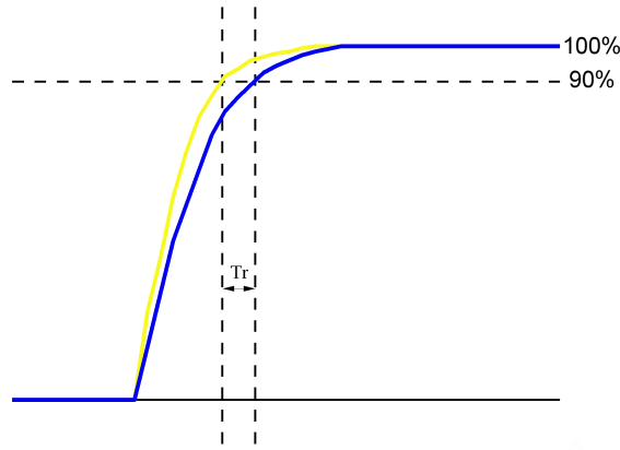
图 2 上升响应时间定义
