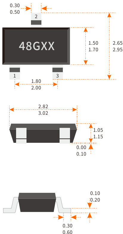
SOT-23 SO封装
