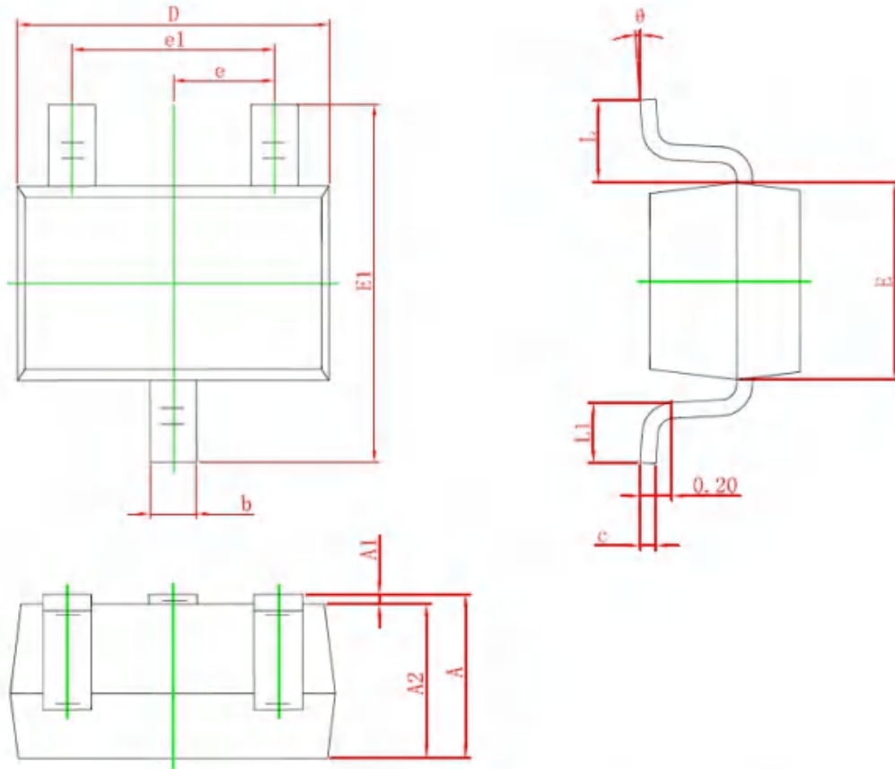
SO (SOT-323)
