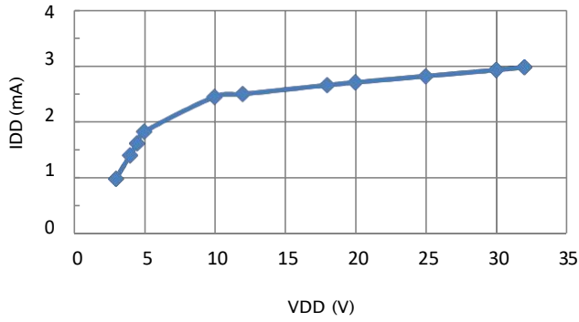
静态电流 vs. 工作电压
